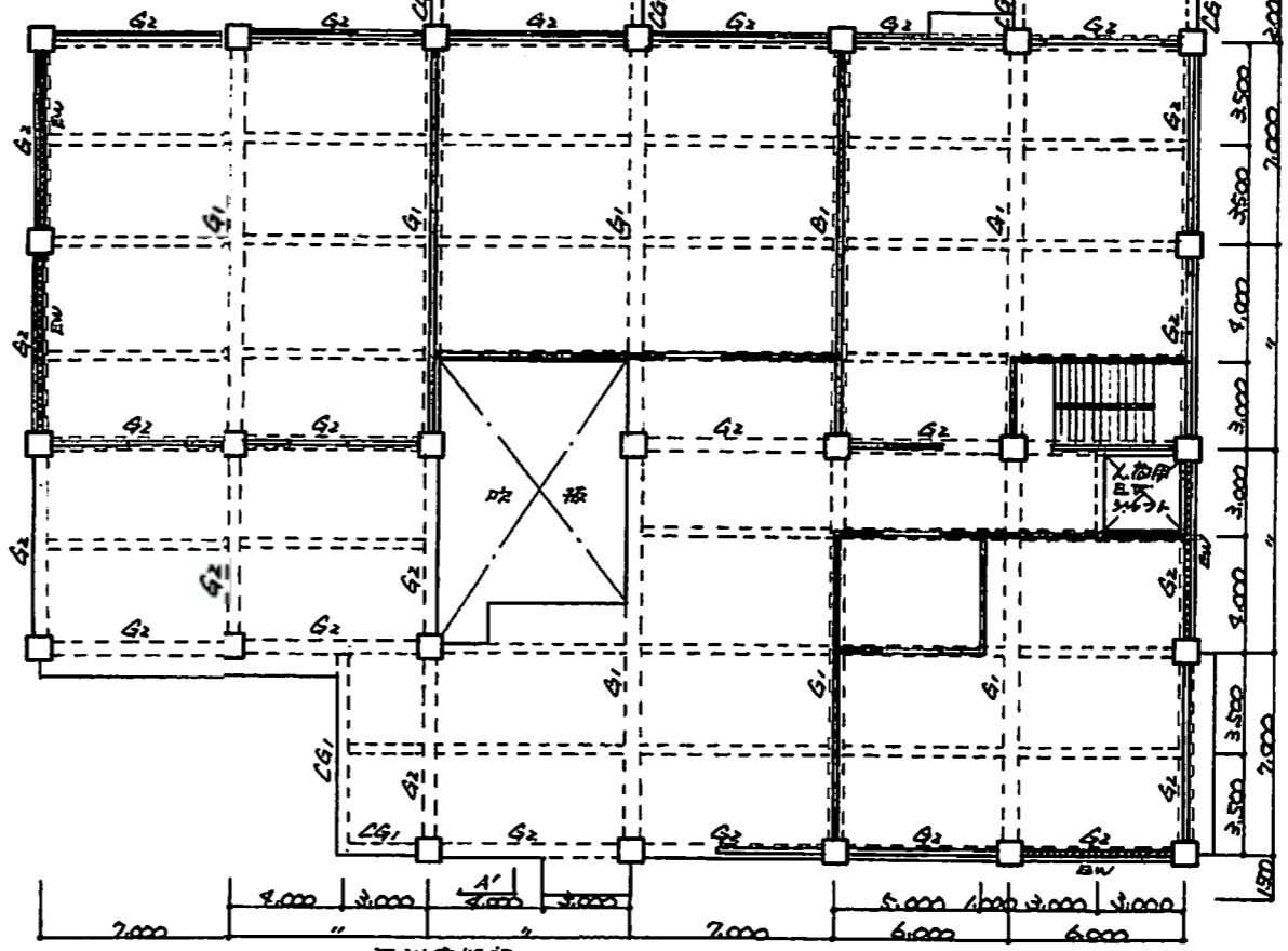
2階梁柱図 S=1/200
