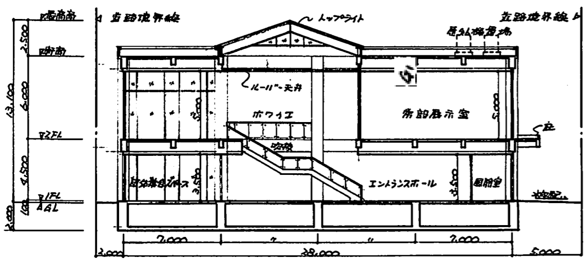
A~A' 断面図 S=1/200
